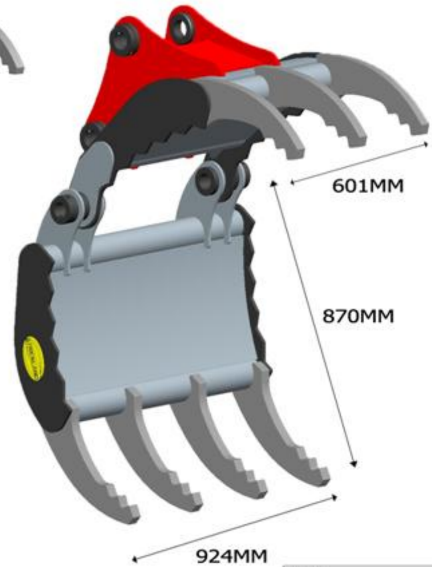
4+3 CONFIGURATION 278KG
